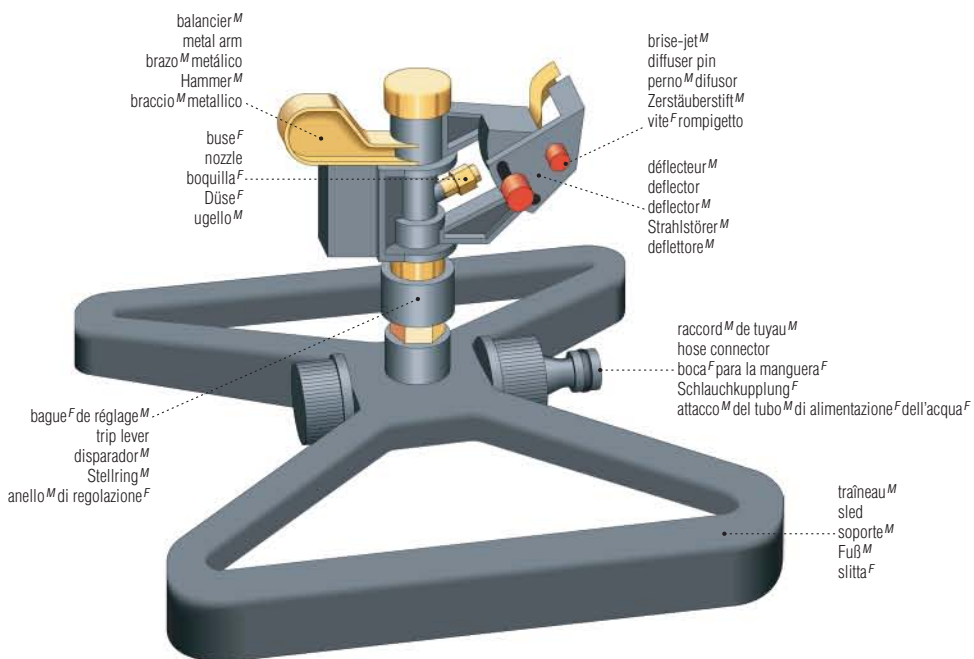
arroiseur M canon M impulse sprinkler irrigador M de impulso M Impulsregner M irrigatore M a impulsi M
